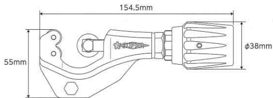
リーマ付チューブカッター TC105R
